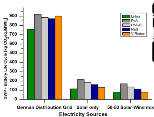
Illustration 11: potentiel de réchauffement global (PRG) de la fabrication et de l'utilisation des types de batterie au lithium-ion (Li-Ion), au plomb-acide (PbA et PbA-R), au sodium-soufre (NaS) et à oxydoréduction au vanadium (V-rédox) par MWh fourni en fonction de l'électricité stockée [source: Hiremath (2015)]
