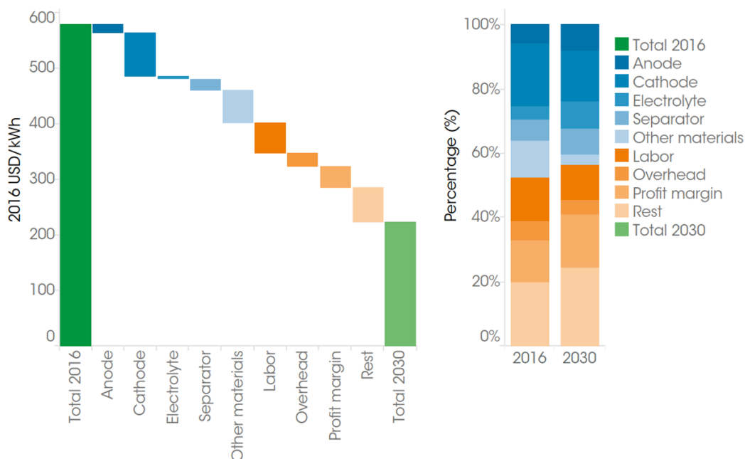
Illustration 32: potentiels de réduction des éléments de coûts des batteries solaires au lithium-ion présentant une composition chimique LFP [source: IRENA (2017)]
