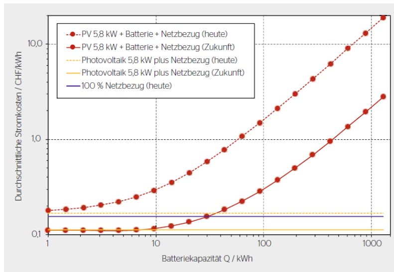
Illustration 33: coûts moyens de revient de l'électricité aux prix actuels et futurs, en fonction de la capacité de la batterie [source: Roth (2018)]
