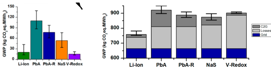
Illustration 10: potentiel de réchauffement global (PRG) des types de batterie au lithium-ion (Li-Ion), au plomb-acide (PbA et PbA-R), au sodium-soufre (NaS) et à oxydoréduction au vanadium (V-rédox) par MWh fourni. À gauche uniquement la fabrication, à droite la fabrication incluant l'utilisation, «C2G» désigne la fabrication, «Losses» les pertes et «Grid» les émissions de l'électricité stockée et fournie [source: Hiremath (2015)]
