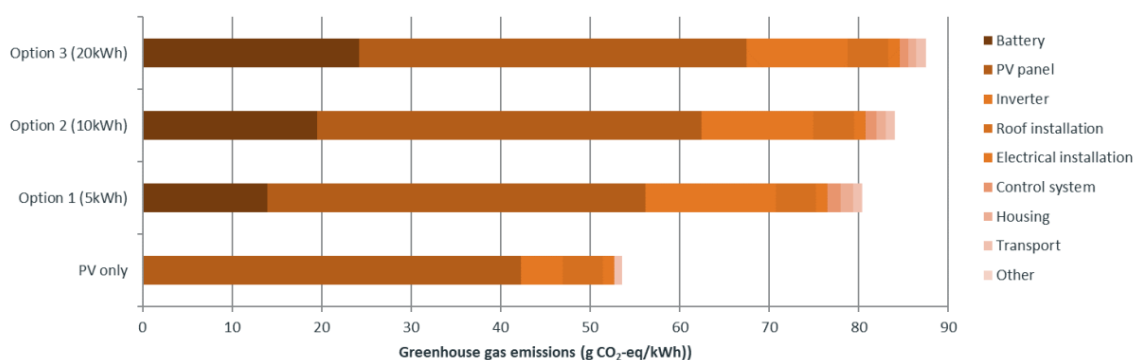
Illustration 13: émissions de gaz à effet de serre du courant d'origine photovoltaïque, si celui-ci est utilisé directement à partir d'une petite installation en toiture «PV seulement» ou stocké provisoirement dans une batterie d'une capacité de 5, 10 ou 20 kWh. [source: Krebs et al. (2020)]
