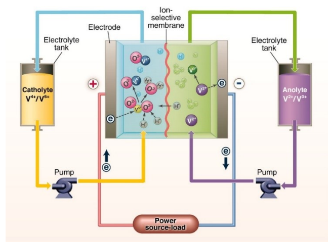
Illustration 5: principe de fonctionnement d'une batterie à oxydoréduction au vanadium [source: Dunn et al. (2011)]
