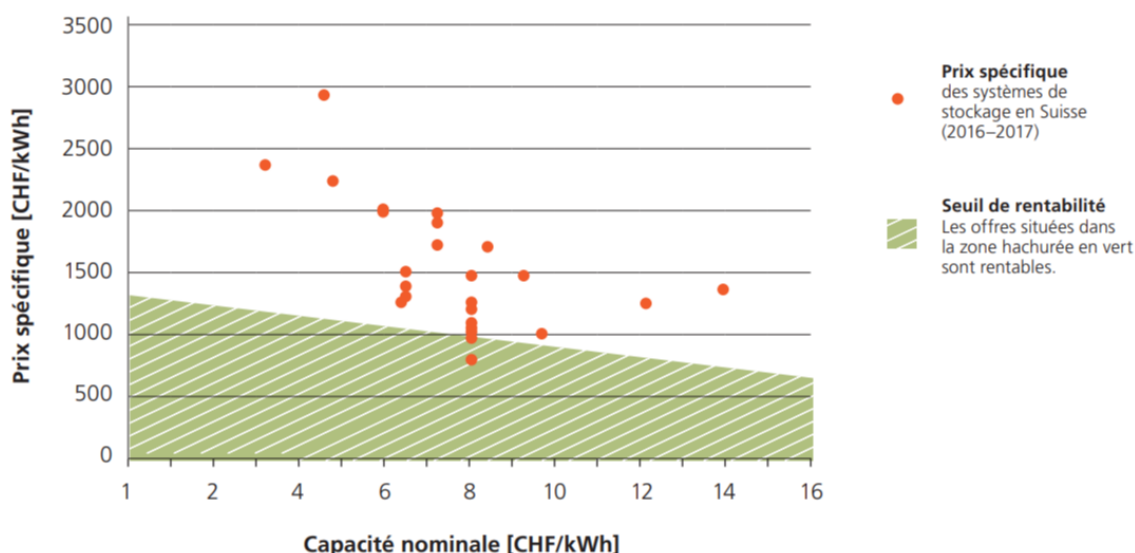
Illustration 19: enquête sur les prix de batteries solaires, frais d'installation compris, en Suisse en 2016-2017 [source: SuisseEnergie (2018)]
