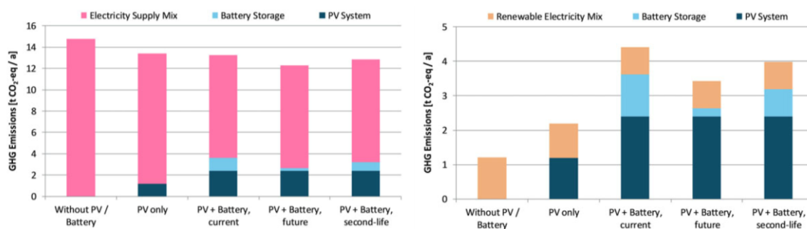
Illustration 9: émissions de gaz à effet de serre de l'alimentation en électricité d'un bâtiment de vestiaires en fonction de l'emploi d'une installation photovoltaïque et de batteries au lithium-ion. Hypothèse quant à l'achat d'électricité: mix de consommation suisse à gauche et mix d'électricité renouvelable dont plus de 95% issus de la force hydraulique à droite [source: Stolz (2019)]
