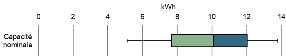
Illustration 24: capacités nominales des batteries solaires sans réserve de secours (n = 26) [source: EBP (2020)]
