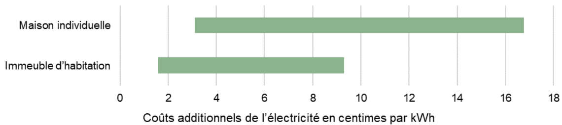
Illustration 36: rentabilité de toutes les combinaisons avec des hypothèses standards: frais supplémentaires par kWh de courant consommé. La valeur à droite de la barre correspond à la «meilleure combinaison» (voir texte), la valeur à gauche à la «plus mauvaise combinaison»
