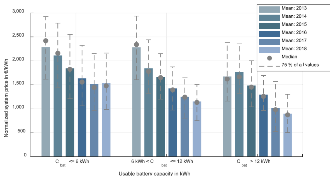
Illustration 30: évolution du prix des batteries solaires au lithium-ion (sans installation) payé par les clients finaux en Allemagne (électronique de puissance et TVA de 19% incluses) [source: Figgenger, (2020)]
