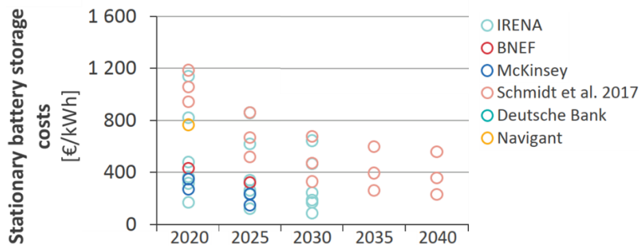
Illustration 31: comparaison des différentes prévisions de coût des batteries solaires sans installation, reposant sur des données bibliographiques (remarque: les estimations de l'IRENA recouvrent toutes les compositions chimiques des batteries au lithium-ion) [source: adaptation de Tsiropoulos, (2020)]
