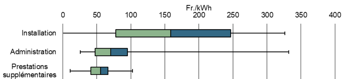
Illustration 28: prix (hors TVA) des composantes de coûts des batteries solaires sans réserve de secours (n = 26) [source: EBP (2020)]
