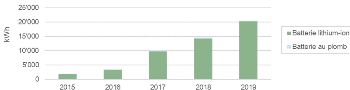
Illustration 17: évolution de la capacité des batteries vendues par an selon la technologie [source: Swissolar (2015), Swissolar (2016) et OFEN (2017-2019)]
