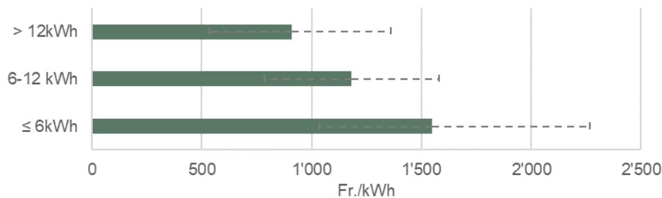
Illustration 20: les prix de batteries solaires payés par les clients finaux allemands en 2018 sans installation (convertis d'euros en francs, déduction de la TVA allemande et TVA suisse en sus) [source des données brutes: Figgenger (2020)]
