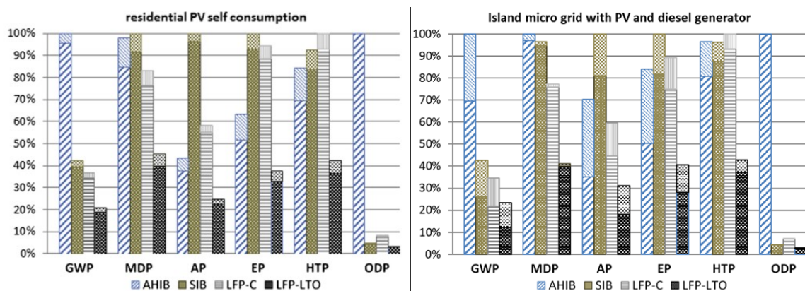
Illustration 12: résultats relatifs du potentiel de réchauffement global (GWP), du potentiel d'épuisement de métaux (MDP), du potentiel d'acidification (AP), du potentiel d'eutrophisation (EP), du potentiel de toxicité humaine (HTP) et du potentiel de destruction de l'ozone (ODP) concernant les types de batterie à eau salée (AHIB), au sodium-ion (SIB), au lithium-fer-phosphate à anode en graphite (LFP-C) et au lithium-fer-phosphate à anode en lithium-titanate (LFP-LTO). Les parties plus sombres des barres reproduisent les impacts induits par la fabrication, les parties claires matérialisant les pertes d'électricité durant l'utilisation [source: Peters & Weil (2017)] 2
