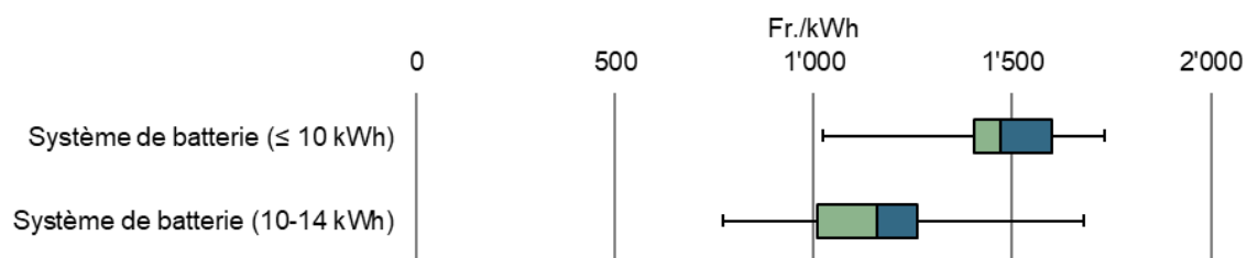
Illustration 26: prix des batteries solaires hors TVA sans réserve de secours (n = 13 [ \leq 10 kWh], m = 13 [ > 10 kWh]) [source: EBP (2020)]
