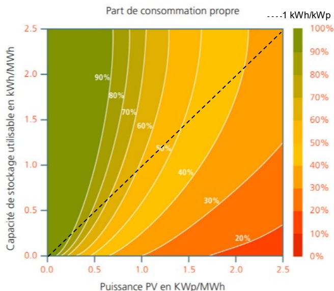
Illustration 34: la part de la consommation propre est calculée au moyen de la puissance photovoltaïque et de la capacité de stockage. Cette évaluation sert de base au calcul de la rentabilité des batteries présenté dans le présent rapport.
