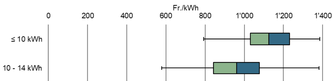
Illustration 27: prix des matériaux (hors TVA) des batteries solaires de tailles différentes sans réserve de secours (n = 13, m = 13) [source: EBP (2020)]
