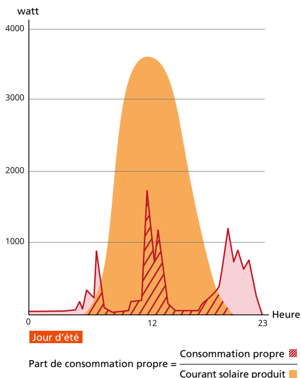
Figure 1: Exemple d'évolution caractéristique de la production de courant solaire quotidienne (source: VESE)
