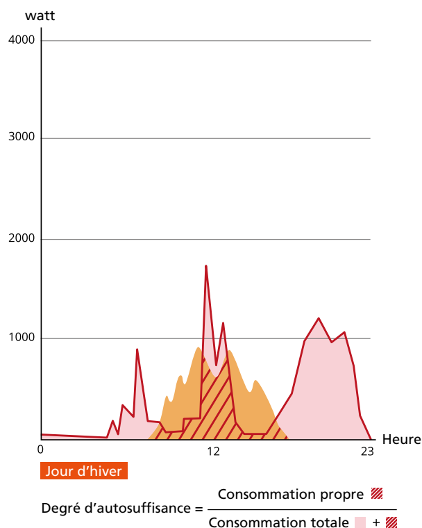
Figure 1: Exemple d'évolution caractéristique de la production de courant solaire quotidienne (source: VESE)
